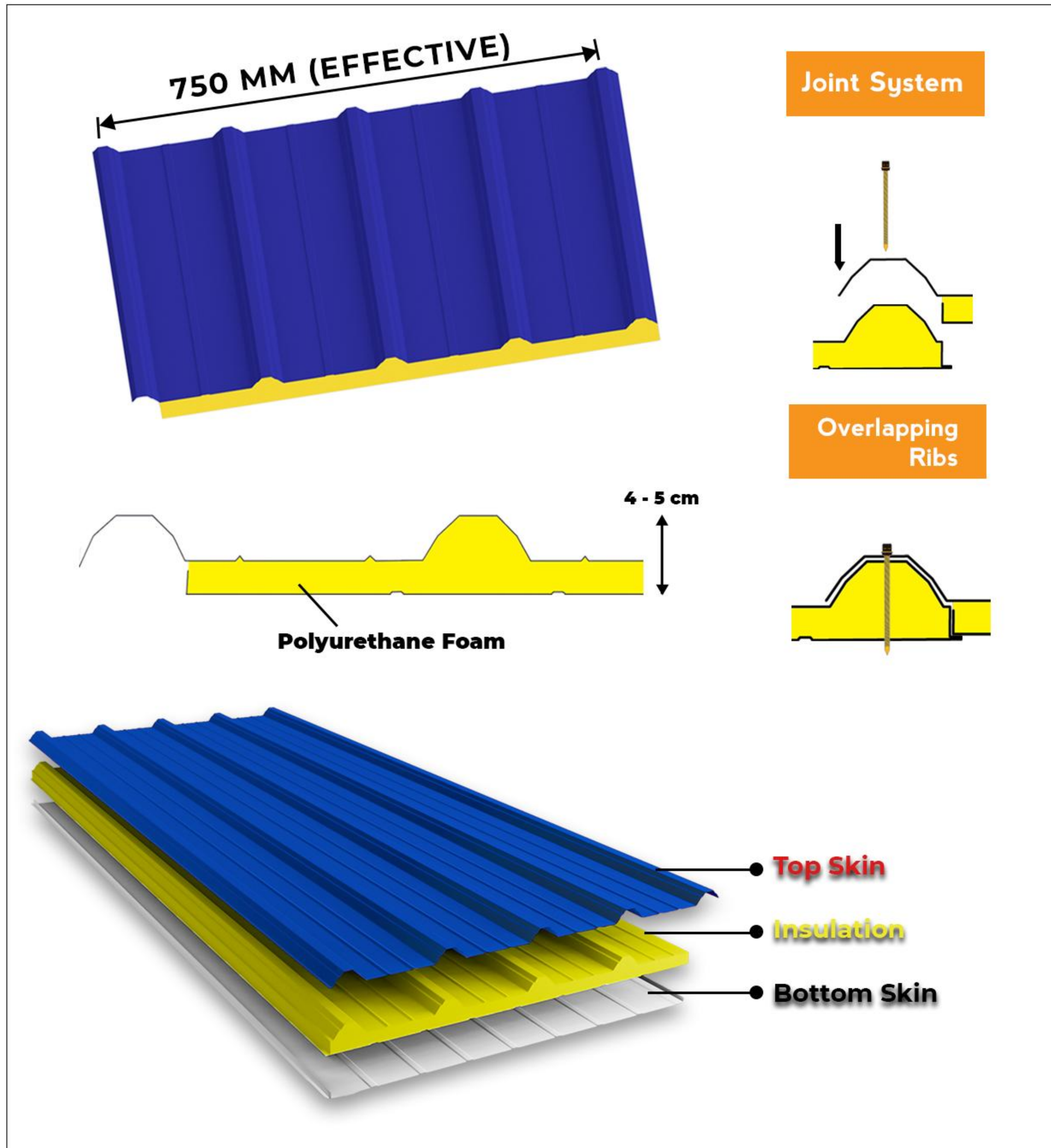
Gambar Teknik ATAP SALJU
