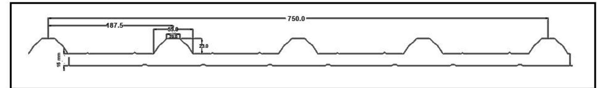
Gambar Teknik ATAP SALJU
