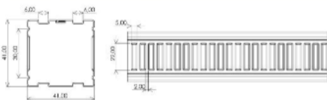
PROFIL HOLLOW 4X4 MAX
