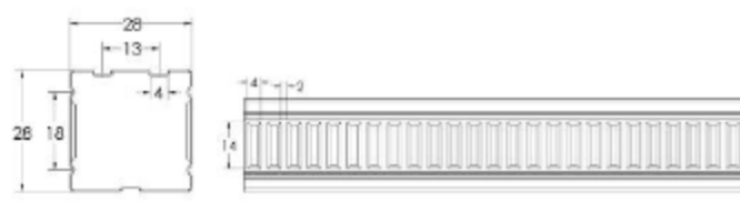
PROFIL HOLLOW 4X4 EVO
