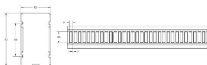
PROFIL HOLLOW 2X4 STD
