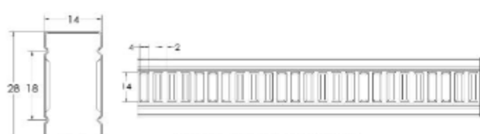
PROFIL HOLLOW 2X4 EVO
