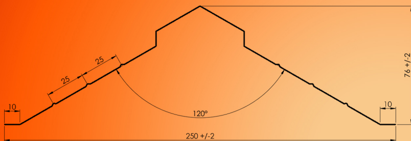
Profil Nok V Minimalis Arjuna
